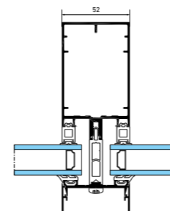
Grille apparente fixe
