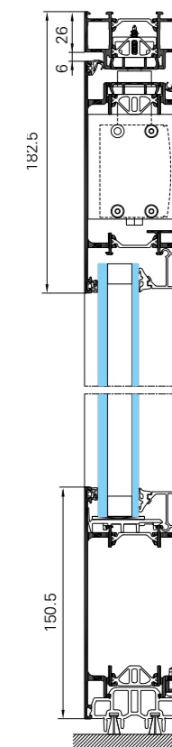
Coupe verticale - Ouverture extérieure
