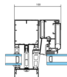
Ouvrant caché à l'italienne
