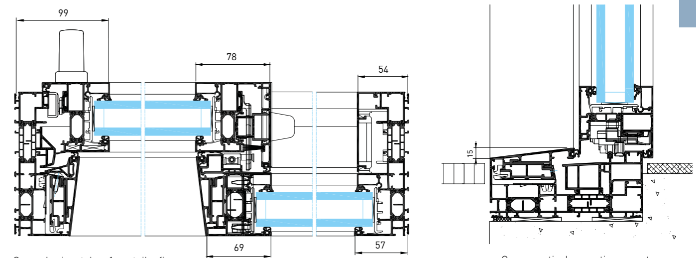
Coupe horizontale - 1 vantail + fixe
