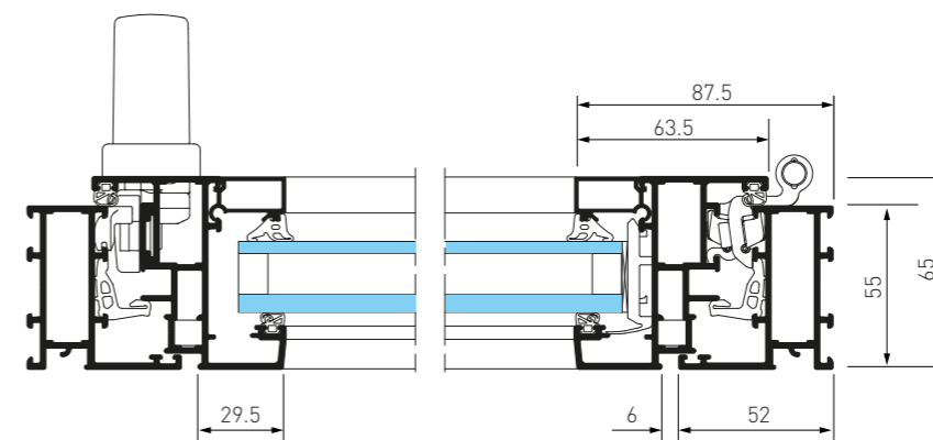
Ouverture intérieure, 1 vantail - coupe horizontale
