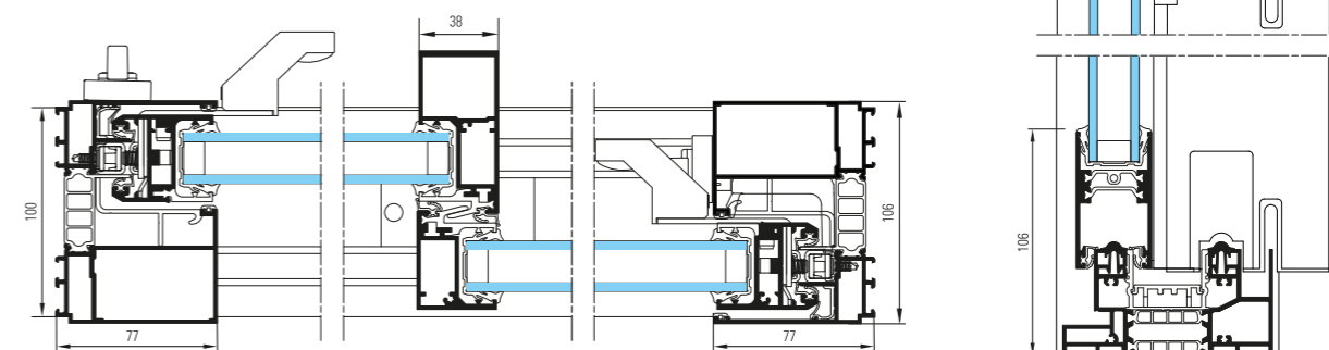
2 vantaux - 2 rails - coupe horizontale
