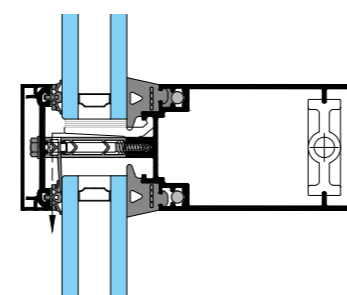
Drainage caché à joint central
