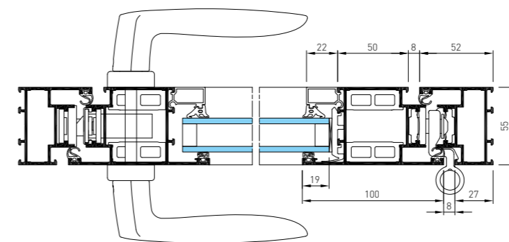
Porte simple action avec plinthe - Coupe horizontale
