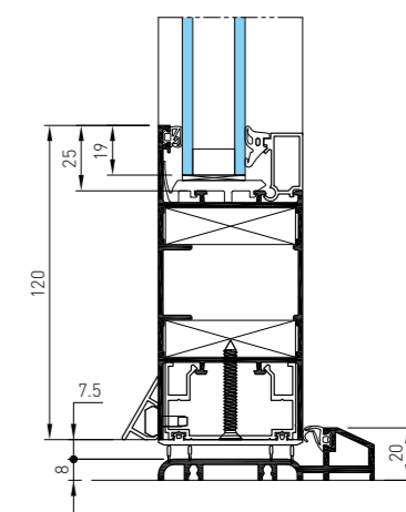
Coupe verticale
