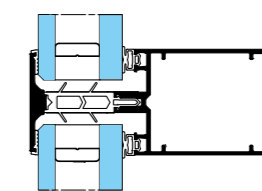
Trame verticale
