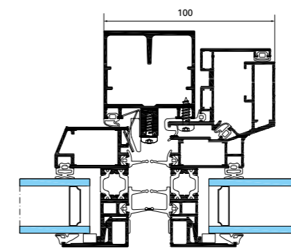
GEODE VEP ouvrant caché à l'italienne
