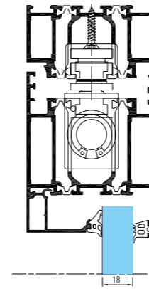
Ferme porte Intégré
