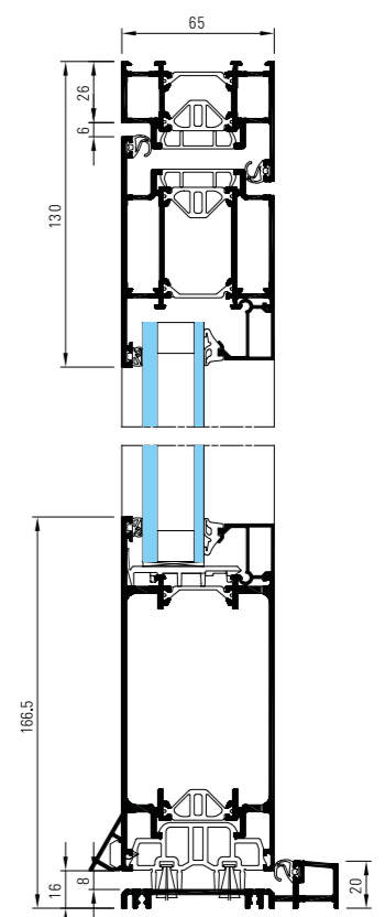
Coupe verticale - Ouverture extérieure
