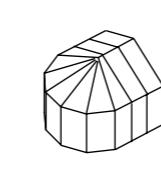
Rayonnante pans coupés à 150°
