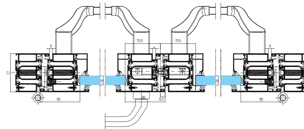
Porte 2 vantaux anti panique ouv. extérieure
