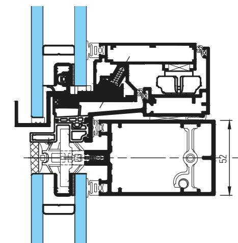
Ouvrant parallèle
