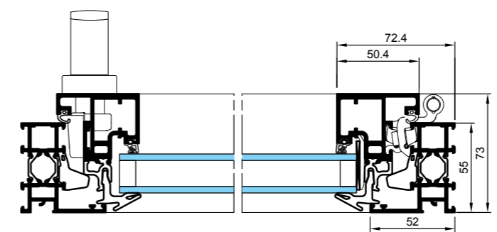
Ouverture intérieure, 1 vantail - Coupe horizontale
