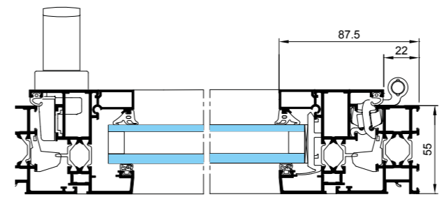
Ouverture intérieure, 1 vantail - Coupe horizontale
