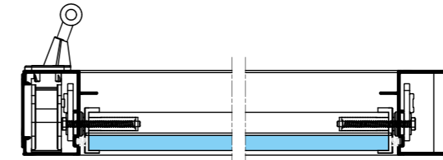
Lame verre - coupe horizontale
