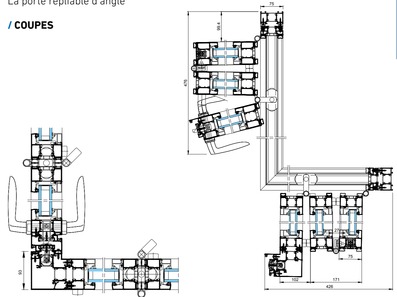
3 x 3 vantaux - ouverture extérieure, angle sortant
