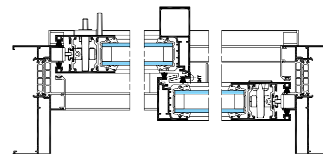
2 vantaux - Monobloc - coupe horizontale
