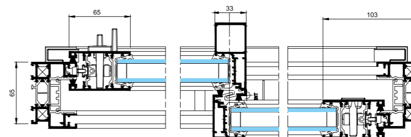
2 vantaux - 2 rails - coupe horizontale
