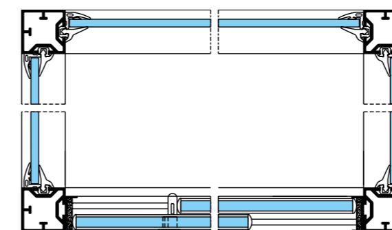
Vitrine avec porte coulissante
