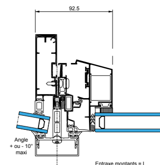
Ouvrant Oscillo-Battant
