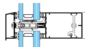
Coupe verticale
