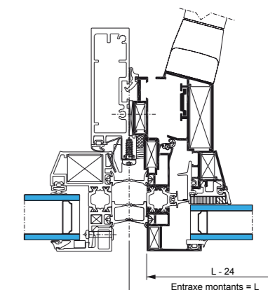
GEODE VEP Oscillo-Battant
