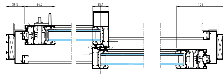
2 vantaux - 2 rails - coupe horizontale
